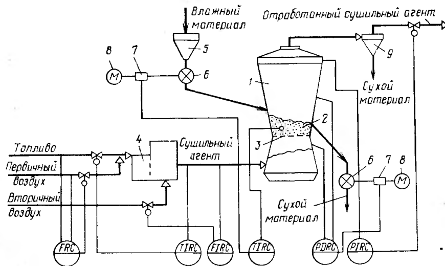
Рисунок А.16 – Схема автоматизации процесса сушки в сушилке с кипящим слоем:
