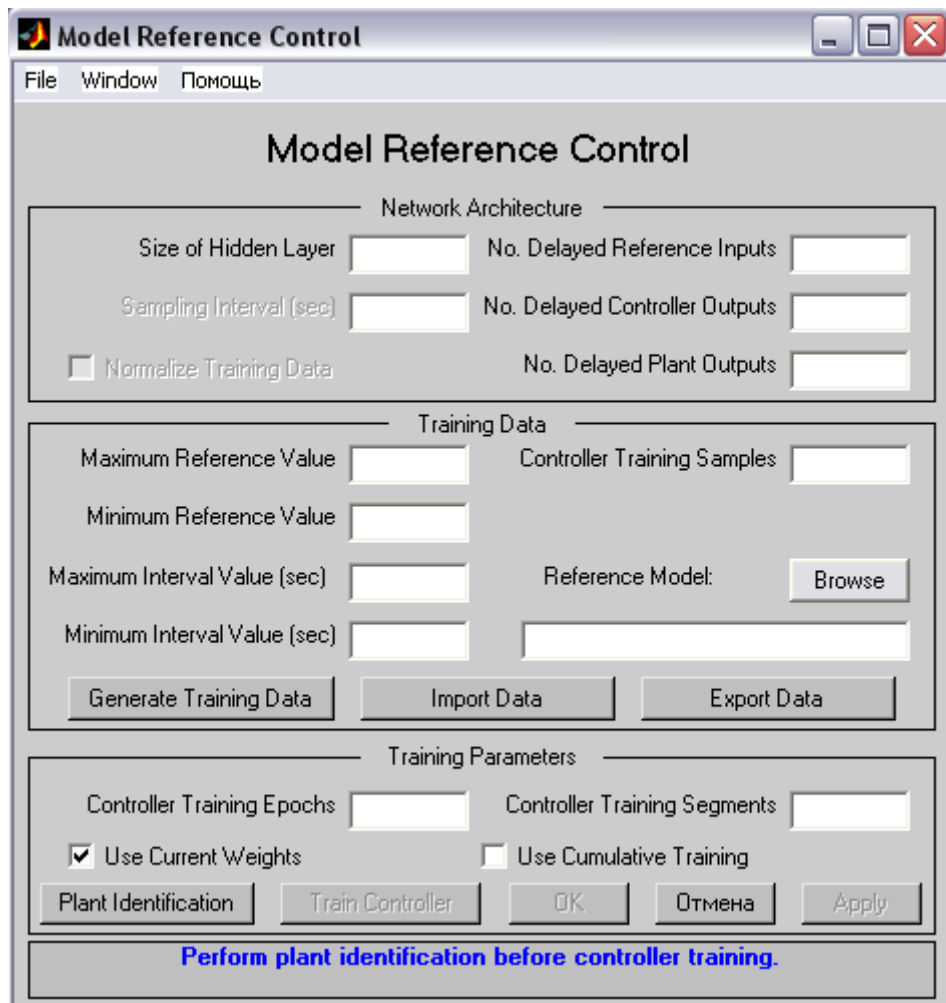
Рис. 10. Настройка процесса обучения управляющей сети
