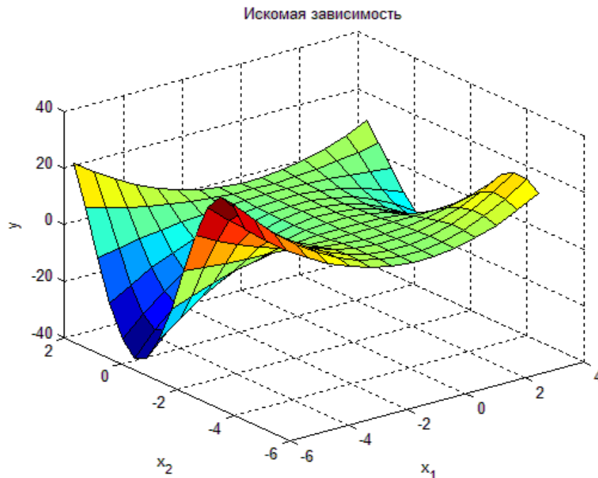
Рис. 1. Графическое представление функции y=x^2 \sin(x2-1)
