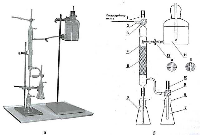
Рисунок 30. Абсорбционная установка:
