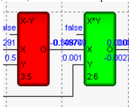
Рис. 40. FBD-диаграмма в режиме отладки
