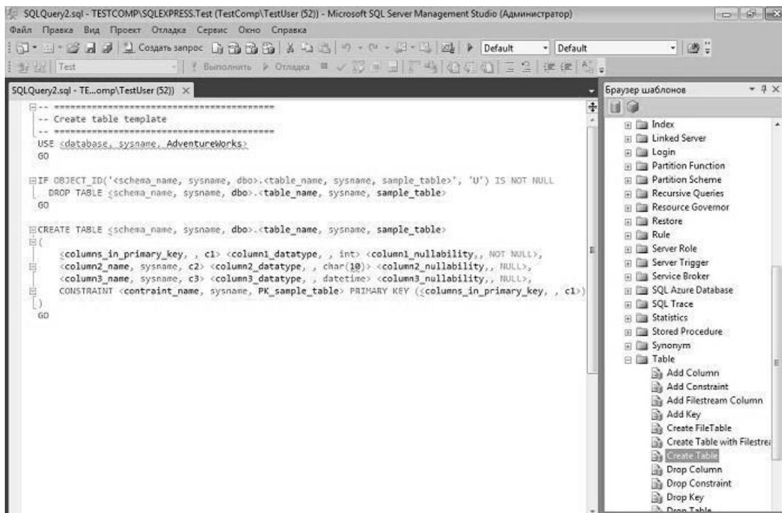
Рис. 5.7. Браузер шаблонов
