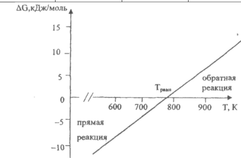
Рисунок 4.1. График зависимости изменения изобарного потенциала от температуры
