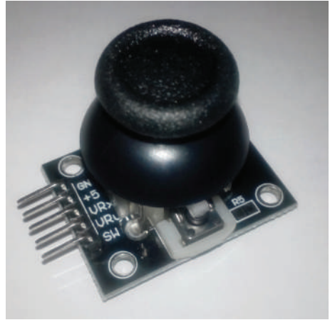
Рис. 33 ❖ Игровой джойстик
