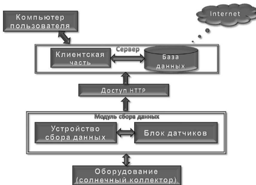
Рис. 5.1. Структурная схема системы сбора и обработки результатов измерений и мониторинга
