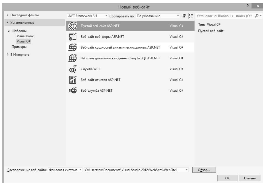
Рис. 6.2. Формирование шаблона
