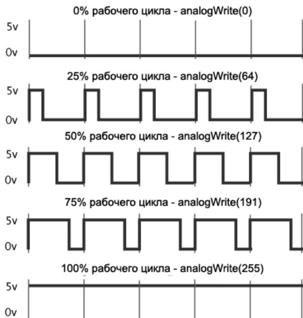
Рис. 2.1. Широтно-импульсная модуляция
