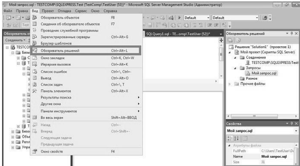
Рис. 5.6. Обзоратель решений
