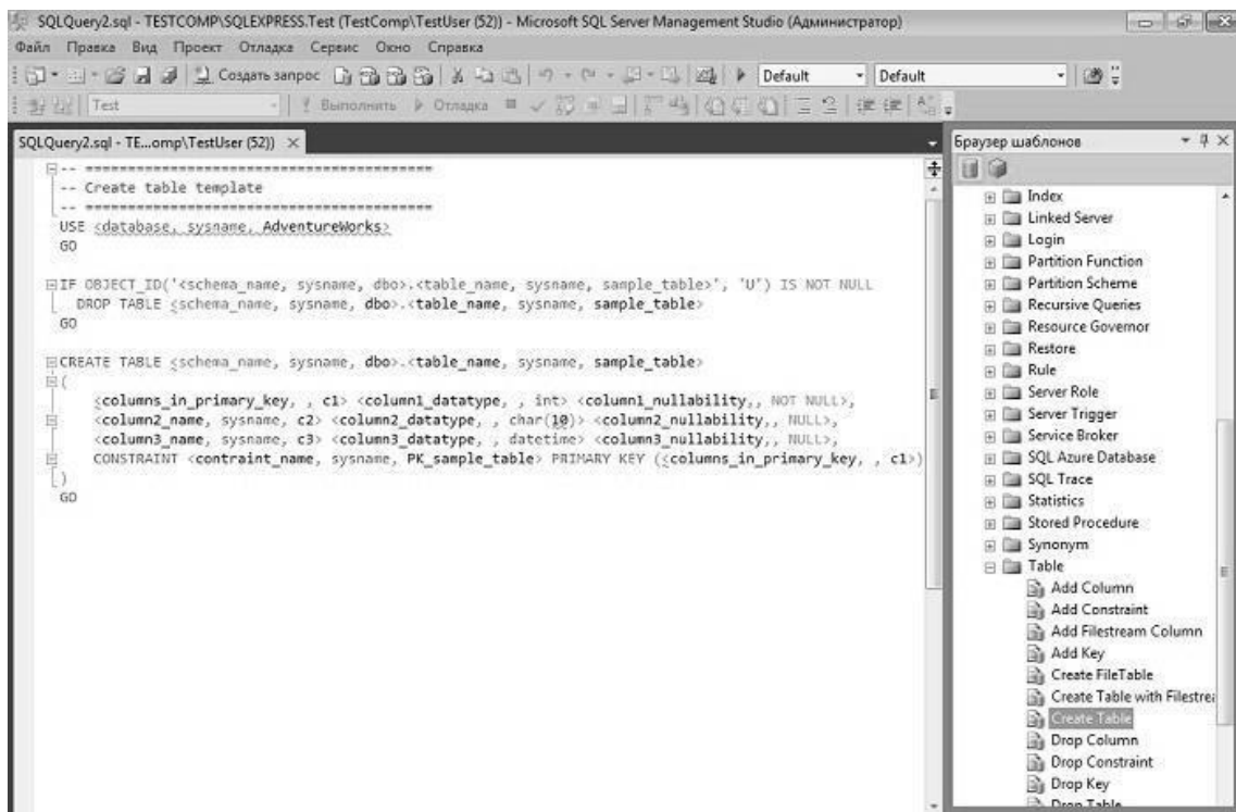
Рис. 5.7. Браузер шаблонов
