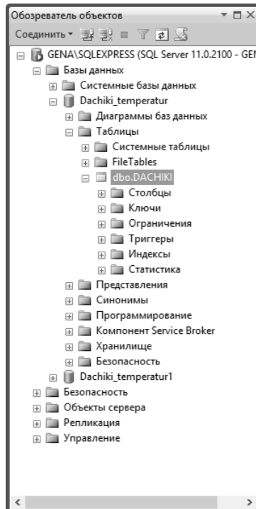
Рис. 5.21. Созданная таблица
