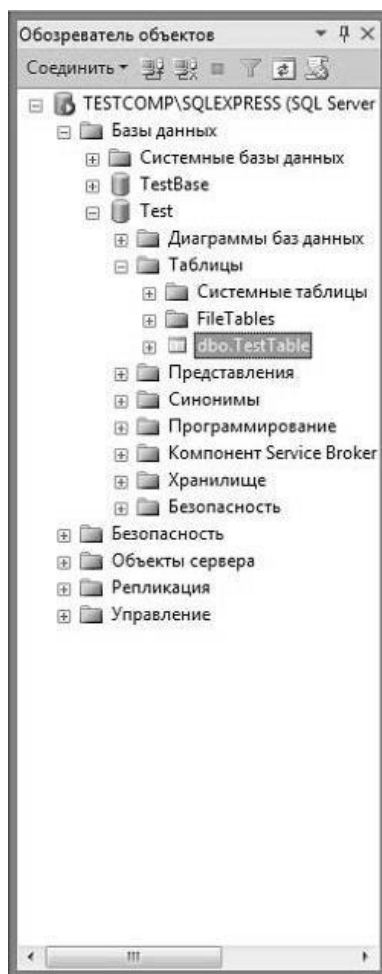
Рис. 5.3. Обозреватель объектов
