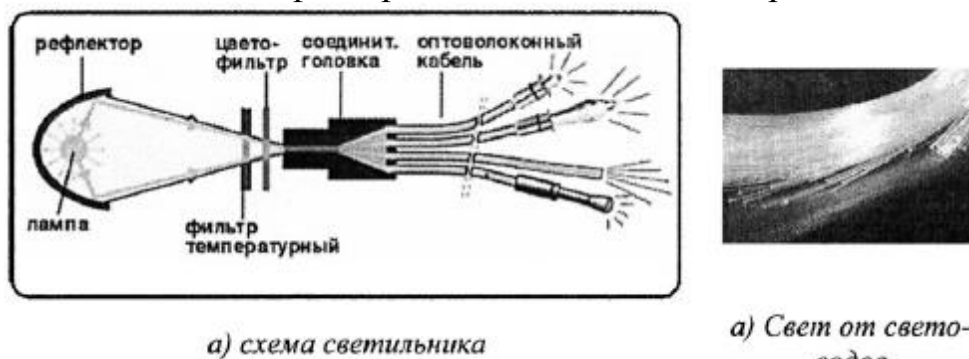
Рис. 1. Декоративный светильник из оптоволоконного кабеля
