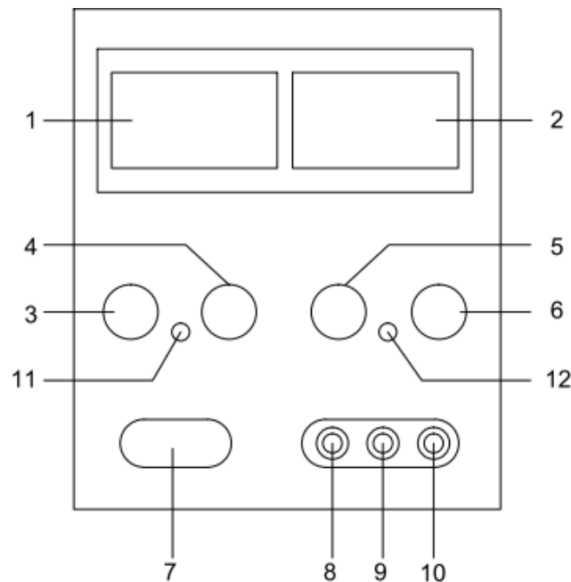
Рис. 2.2. Передняя панель прибора НУ 3005:
