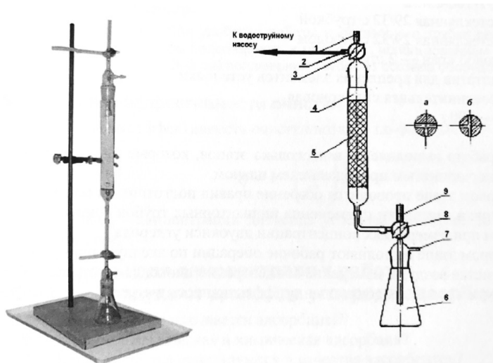
Рисунок 32. Адсорбционная установка:
