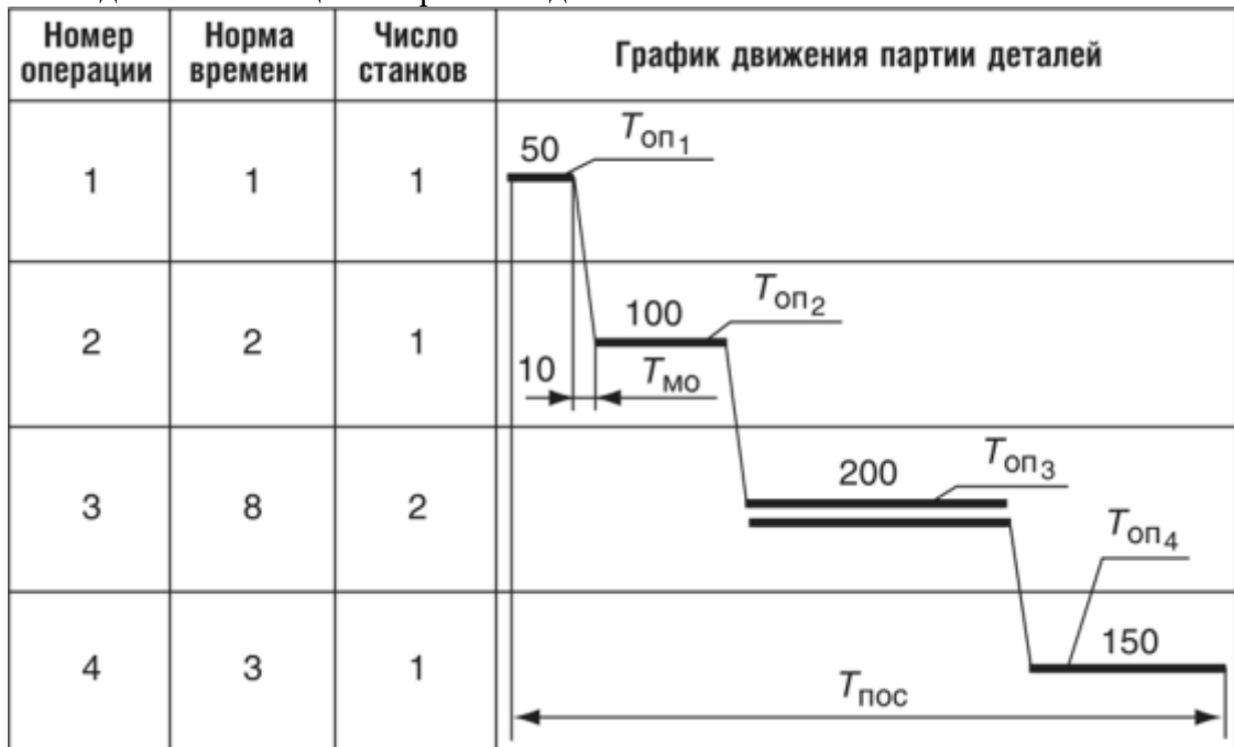
Рис. Последовательный цикл обработки деталей
