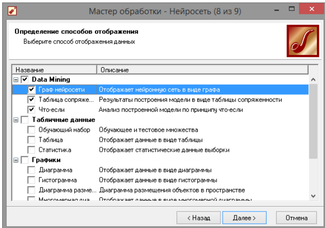
Рис. 2.19 - Визуализаторы
