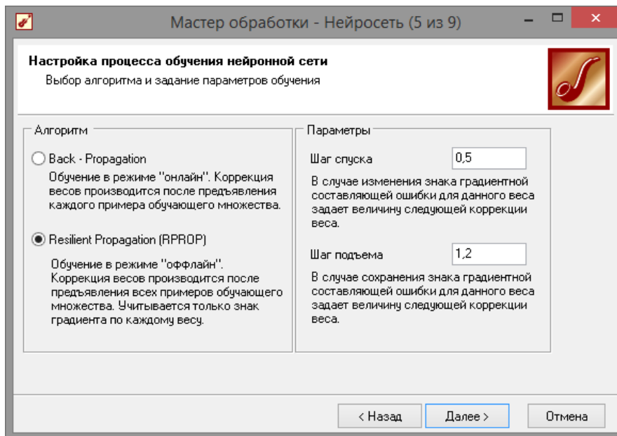
Рис. 3.5 - Алгоритм обучения
