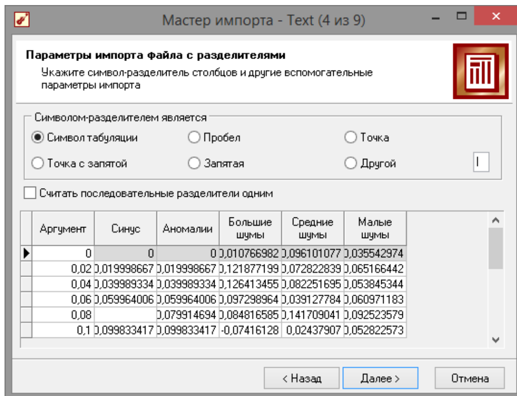
Рис. 1.5 - Параметры разделителей
