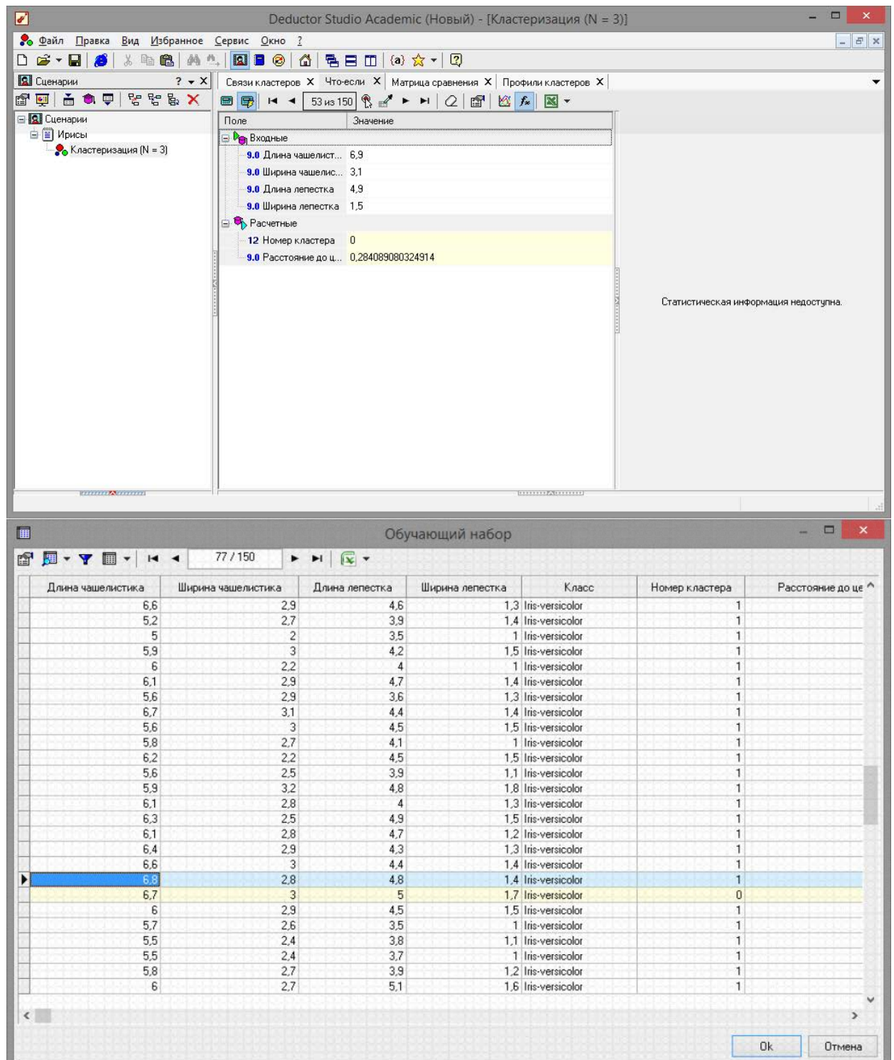
Рис. 2.10 - Инструмент «Что-Если»
