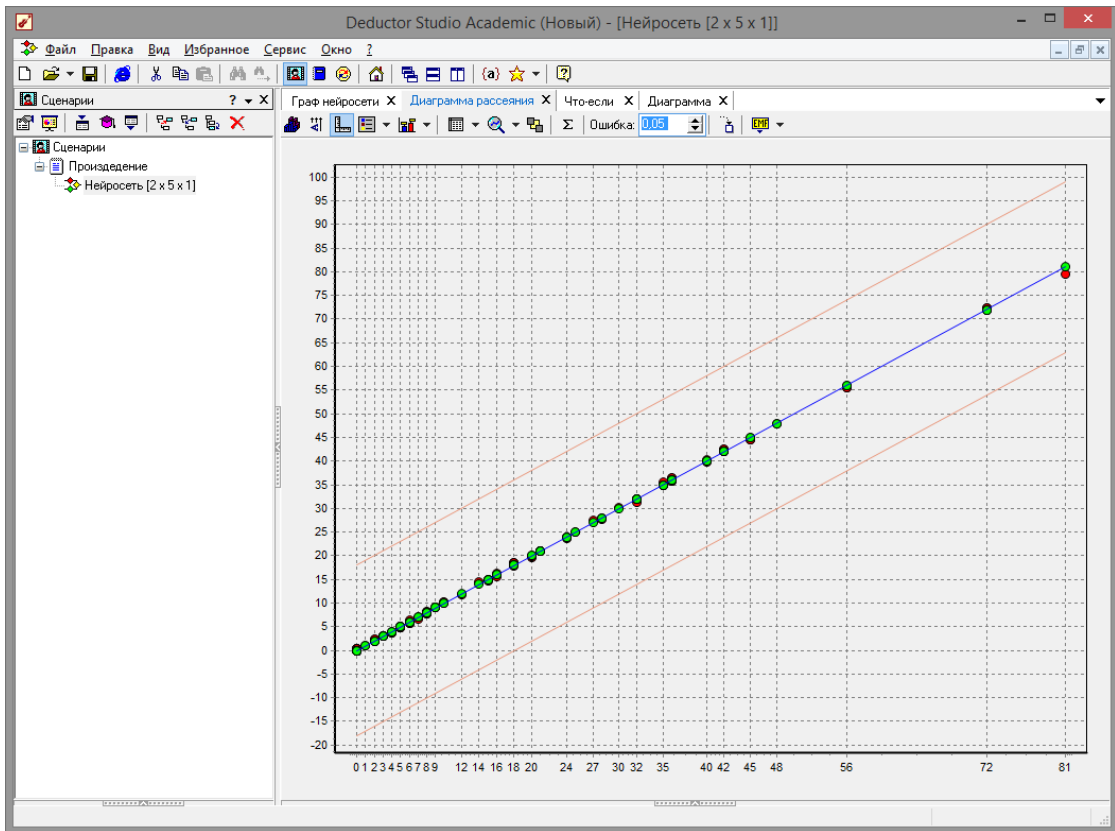
Рис. 3.9 - Диаграмма рассеяния
