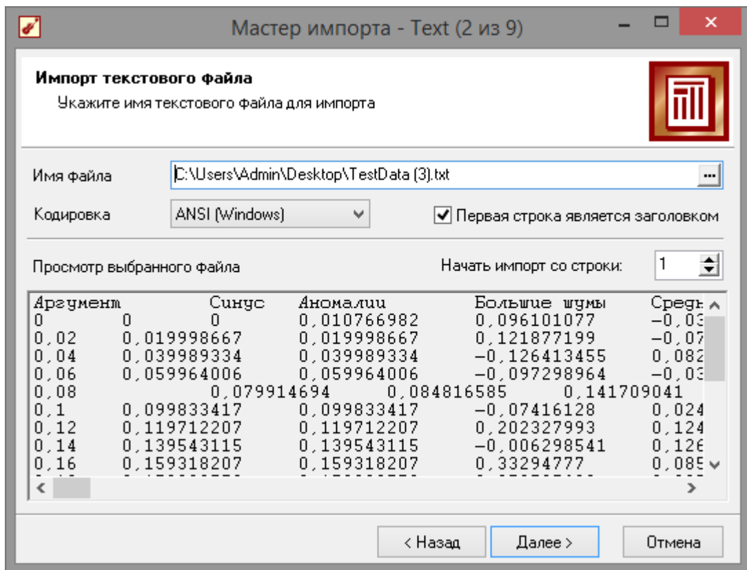
Рис. 1.3 - Выбор файла
