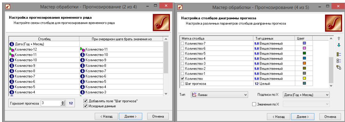
Рис. 3.25 - Мастер прогнозирования
