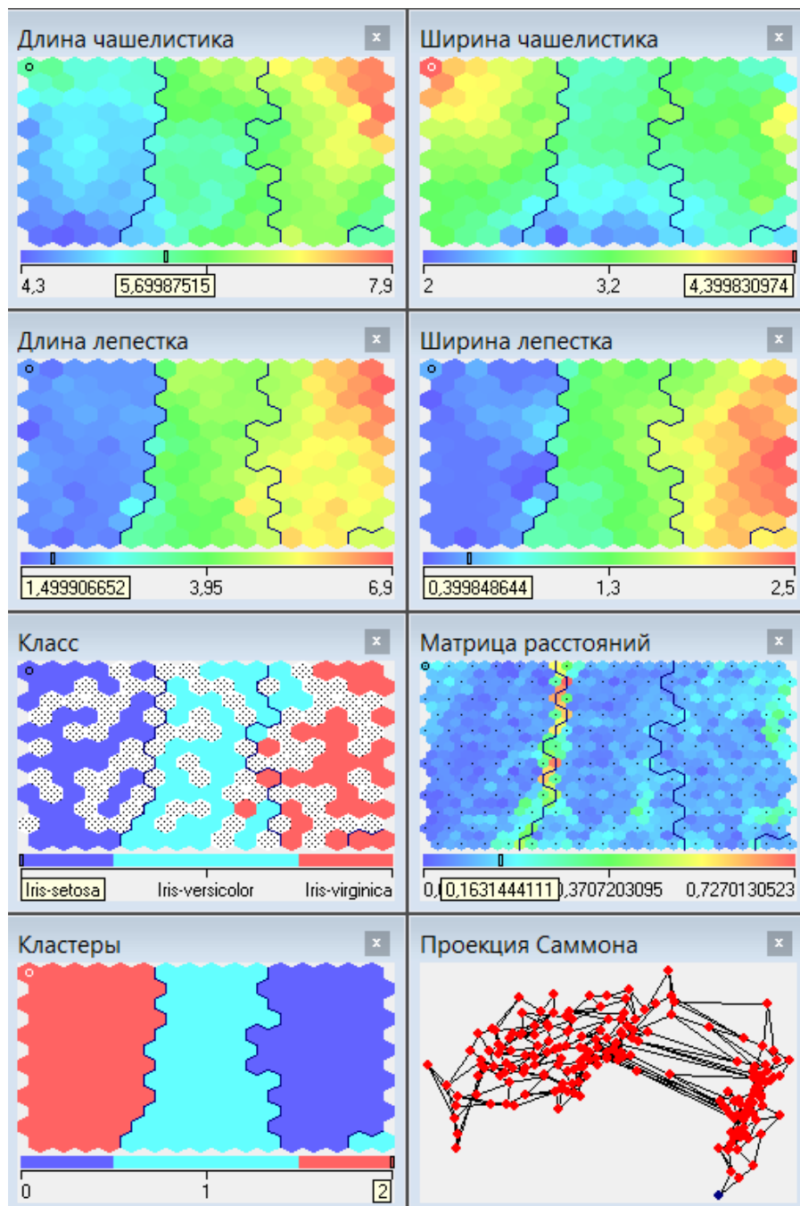
Рис. 4.11 - Карта Кохонена
