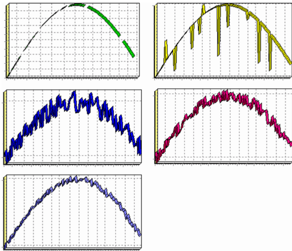
Рисунок 1.12 - Варианты столбцов
