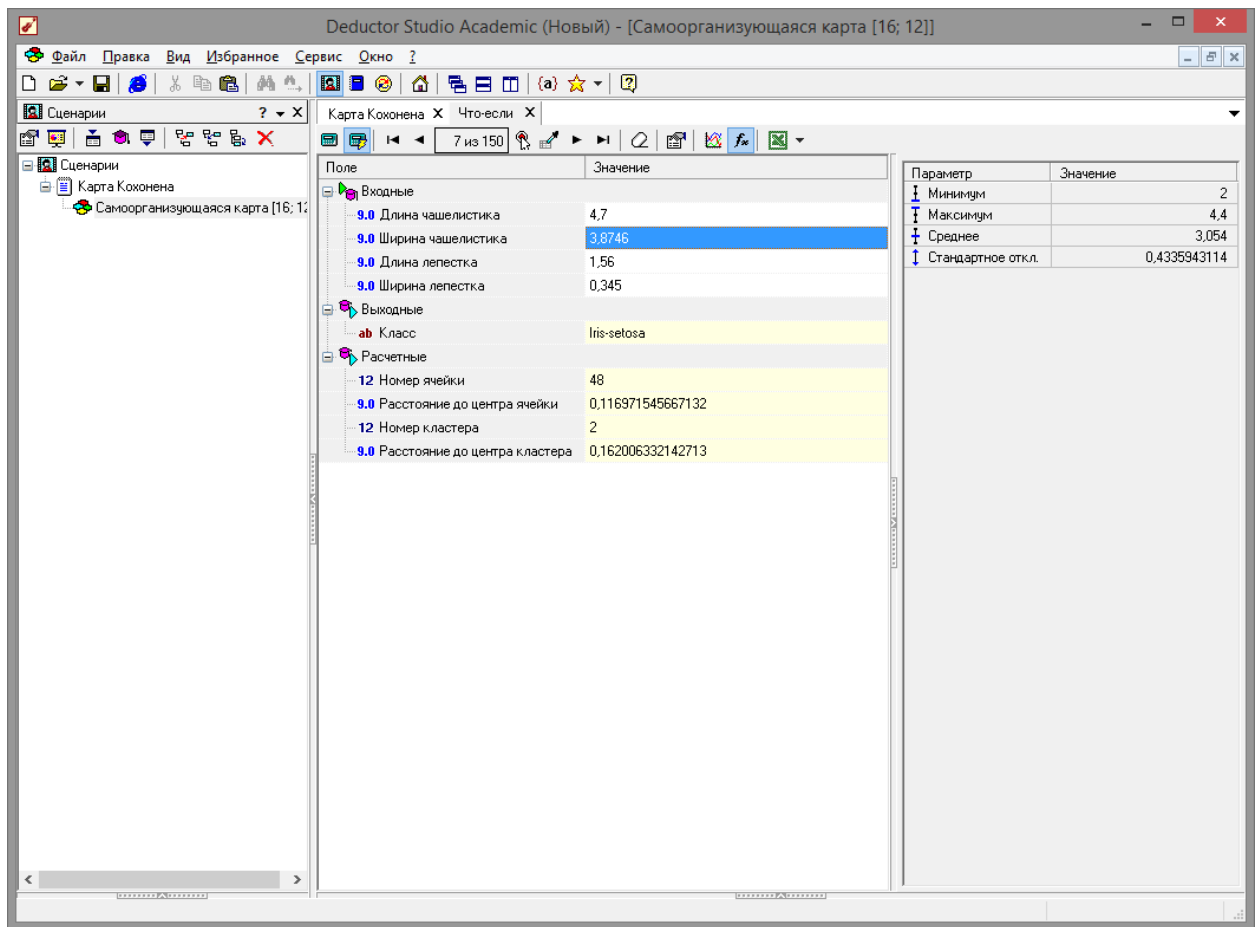
Рис. 4.12 - Таблица «Что-Если»
