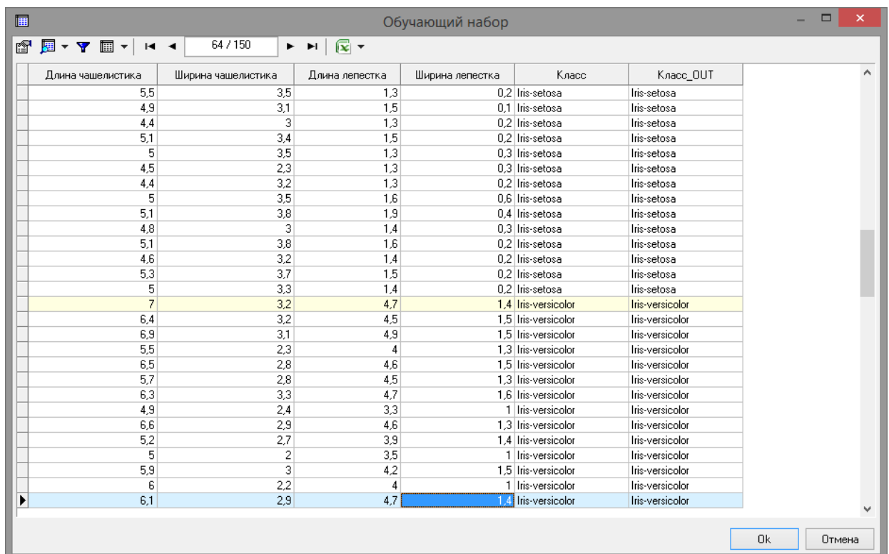
Рис. 2.22 - Инструмент «Что-Если»
