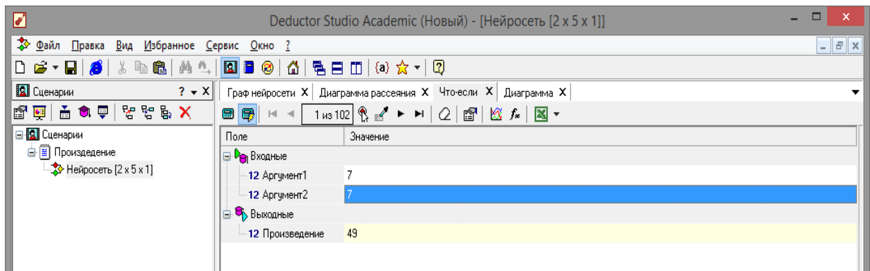
Рис. 3.11 - Инструмент «Что-Если»
