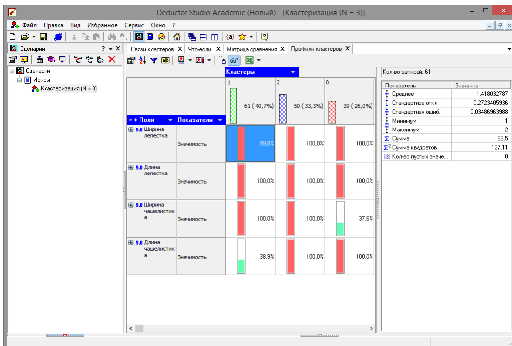
Рис. 2.8 - Профили кластеров
