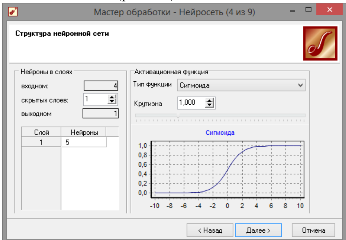
Рис. 2.15 - Параметры обучения
