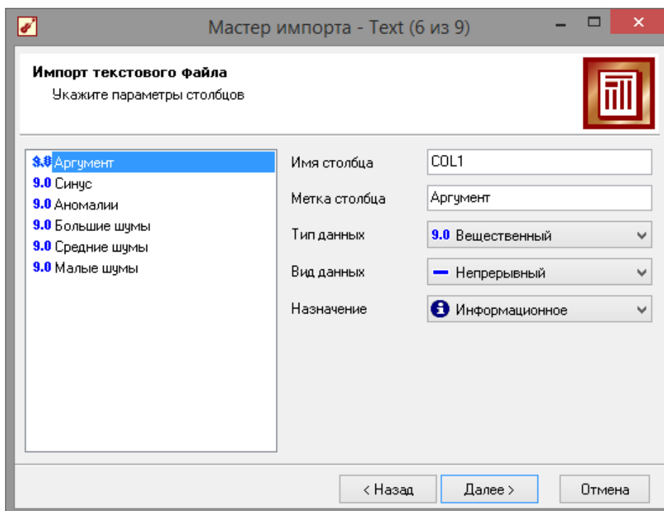
Рис. 1.6 - Параметры столбцов
