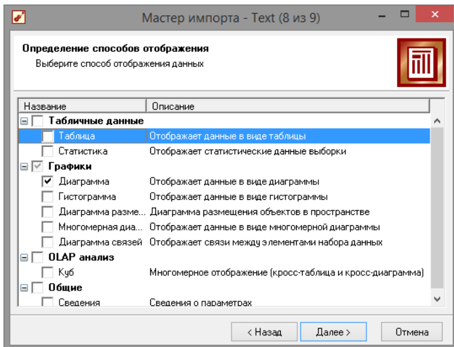
Рис. 1.8 - Способ отображения
