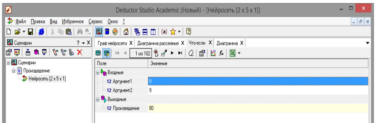
Рис. 3.12 - Ошибки прогнозирования
