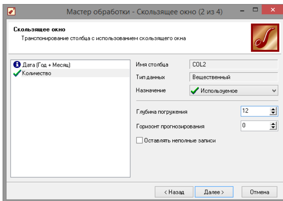
Рис. 3.17 - Скользящее окно
