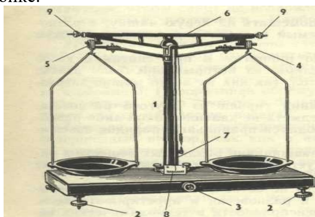
Рис. 2. Теххимические весы: 1 — стойка весов; 2 — установочный винт; 3 — маховичек; 4 — стремя; 5 — призма; 6 — коромысло; 7 — стрелка; 8 — шкала; 9 — грузики.
