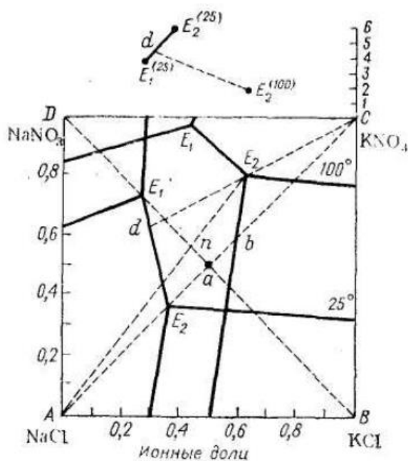
Рисунок 5.1 –Изотерма растворимости в системе \text{NaNO}_3 - \text{KCl} - \text{H}_2\text{O} при 100 и 25^\circ\text{C}
