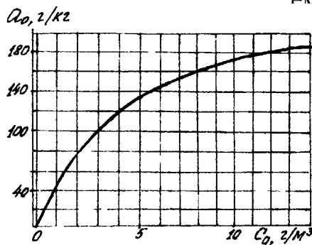
Рис. 2.1. Изотерма паров этилового спирта на активированном угле при 20°C
