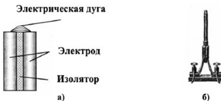
Рис. 4. Свеча Яблочкова
