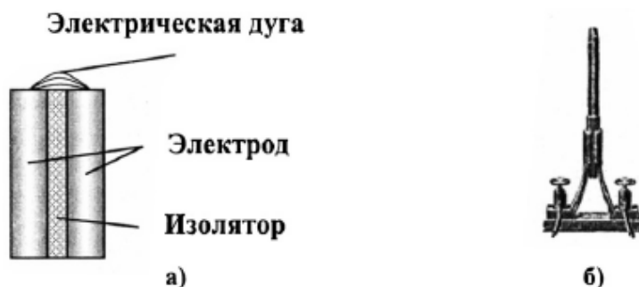
Рис. 4. Свеча Яблочкова
