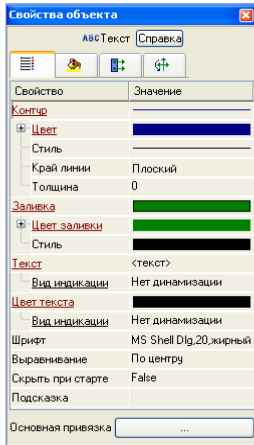
Рис. 31. Задание статических атрибутов текста
