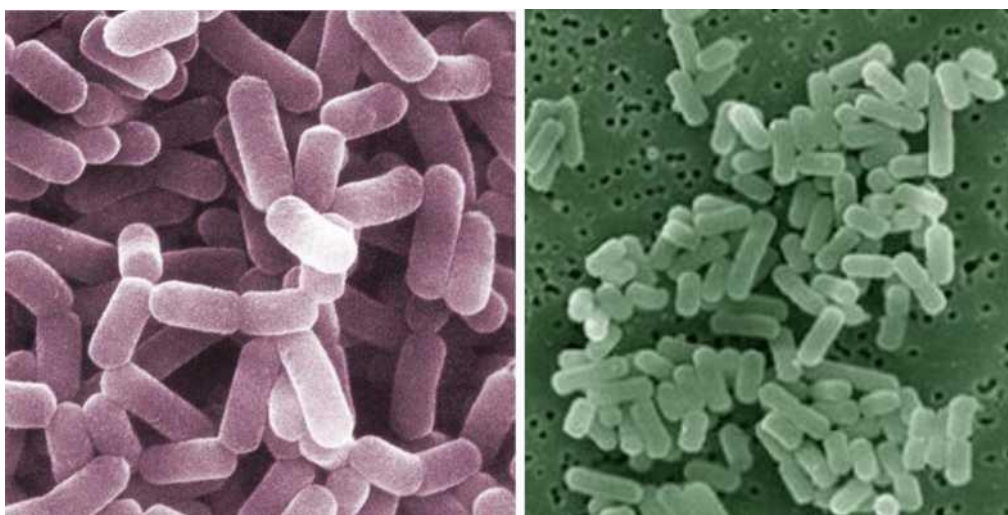
Рис. 11. Стрептобактерии:
