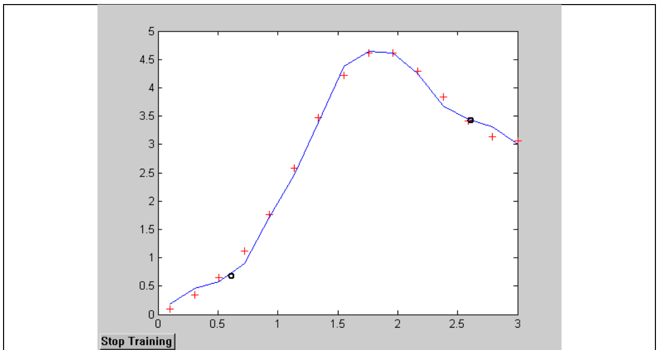
Рис. 4. Результаты моделирования сети: + - исходные данные; сплошная линия и символ «o» – результаты моделирования всей зависимости и в контрольных точках
