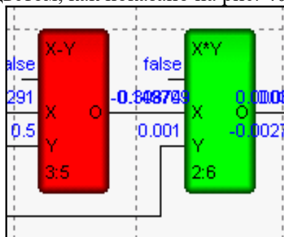
Рис. 40. FBD-диаграмма в режиме отладки
