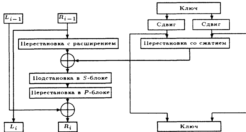
Рисунок 3.8 – Один цикл DES-преобразования
