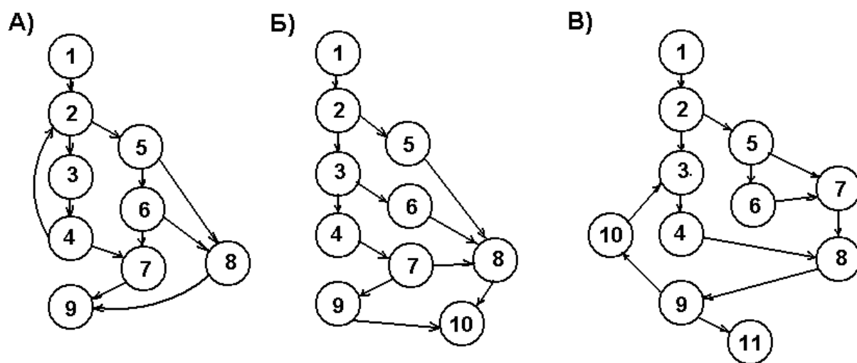
Рис. 4.4. Потоковые графы
