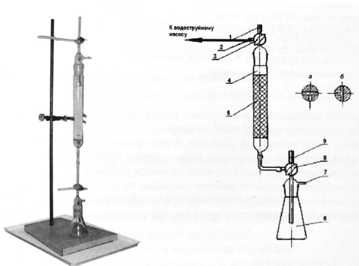
Рисунок 32. Адсорбционная установка: а – установка в собранном виде на штативе; б – схема установки.
