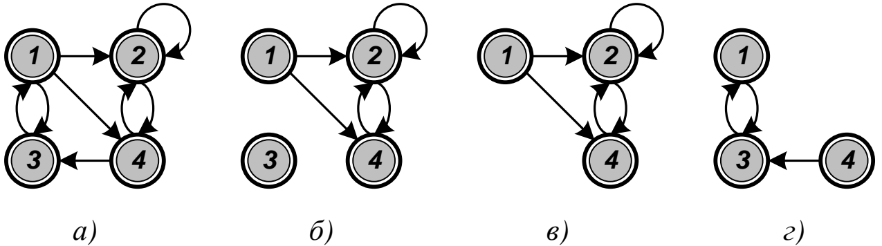
Рисунок 4.2 — Граф и его части: а) исходный граф; б) суграф; в) подграф; г) дополнение подграфа
