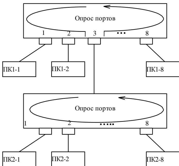
Рис. 3.3 Архитектура сети 100VG AnyLAN
