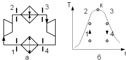
Рис. 7.1. Машина Карно: а – конструкция; б – цикл
