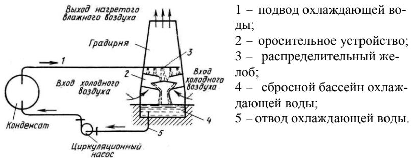
Рис. 2.4. Испарительная градирня
