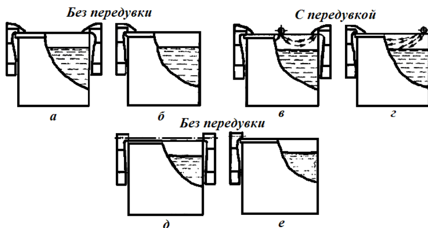
Рисунок 1 – Схемы бортовых отсосов: опрокинутые (а, в - двубортовые; б, г - однобортовые); обычные (д - двубортовый; е - однобортный)
