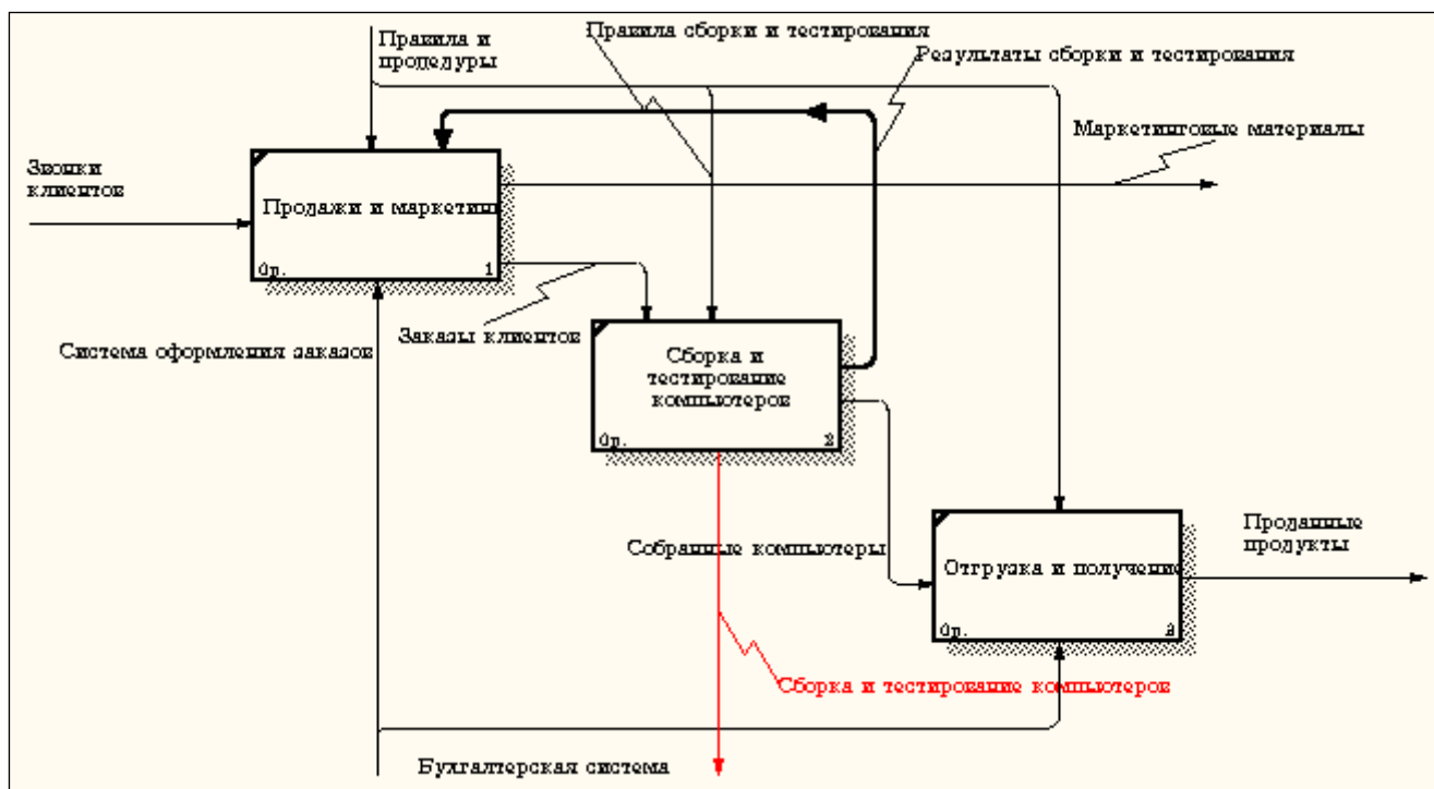
Рисунок 6.4 – На диаграмме А0 модели "Деятельность компании" Появилась стрелка вызова "Сборка и тестирование компьютеров"
