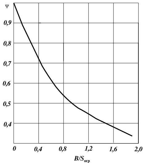
Рисунок 1 – Зависимость коэффициента диффузности \psi от постоянной помещения V и площади ограждения S_{огр}
