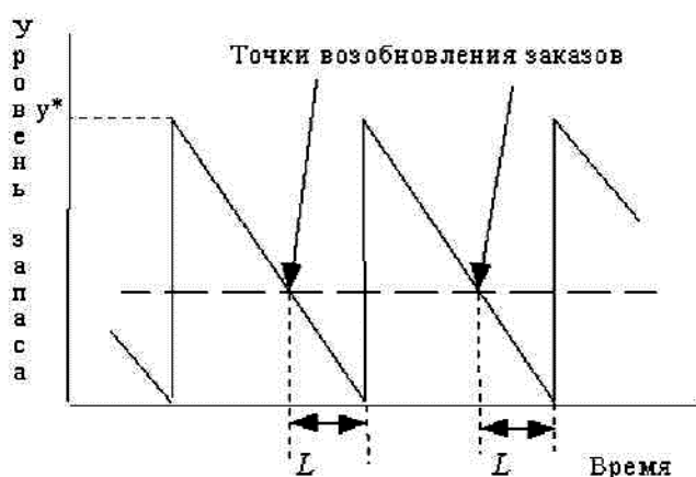
Рисунок 3 — Точка возобновления заказа опережает ожидаемую поставку
