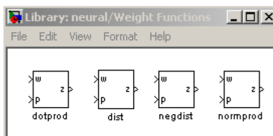
Рис. 4. Библиотека блоков весовых коэффициентов
