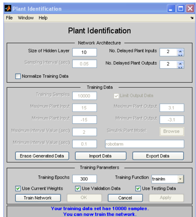
Рис. 19. Модифицированное окно для построения модели ОУ
