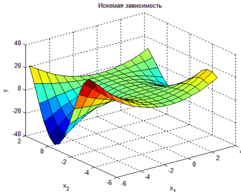
Рис. 1. Графическое представление функции y = x_1^2 \sin(x_2 - 1)
