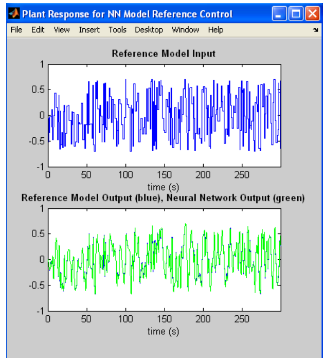
Рис. 23. Выход эталонной модели и объекта управления
