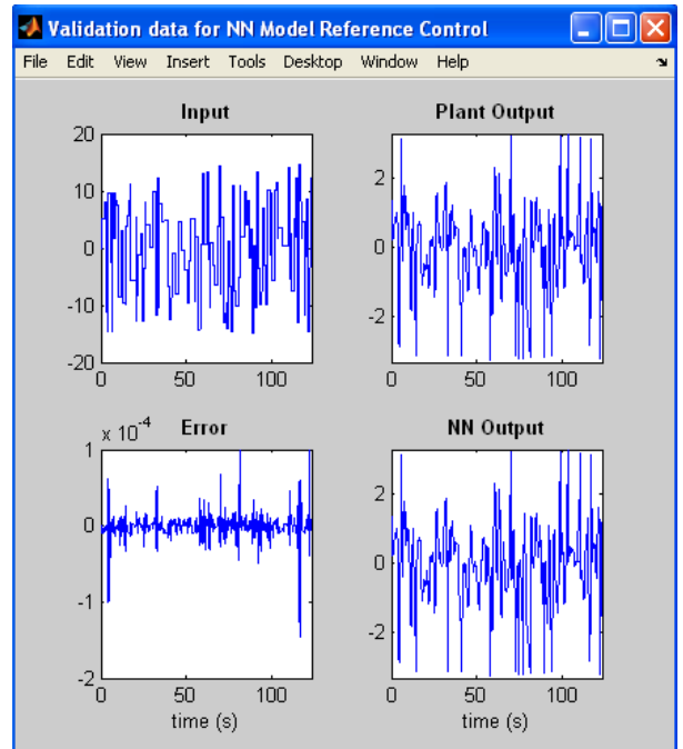
Рис. 21. Результат тестирования модели на контрольном множестве
