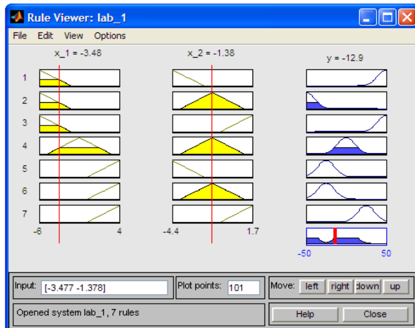
Рис. 5. Визуализация нечеткого вывода Mamdani
