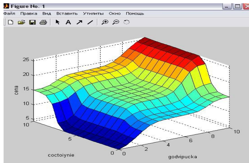
Рис.5.2. Результат выполнения функции gensurf (имя)
