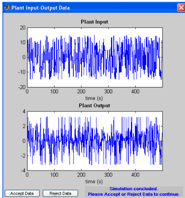
Рис. 18. Сигнал ОУ в режиме его идентификации
