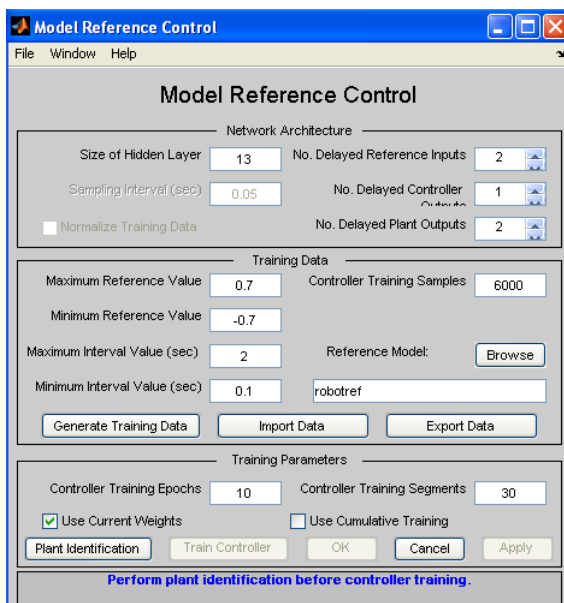
Рис. 16. Окно настроек нейросетевых моделей
