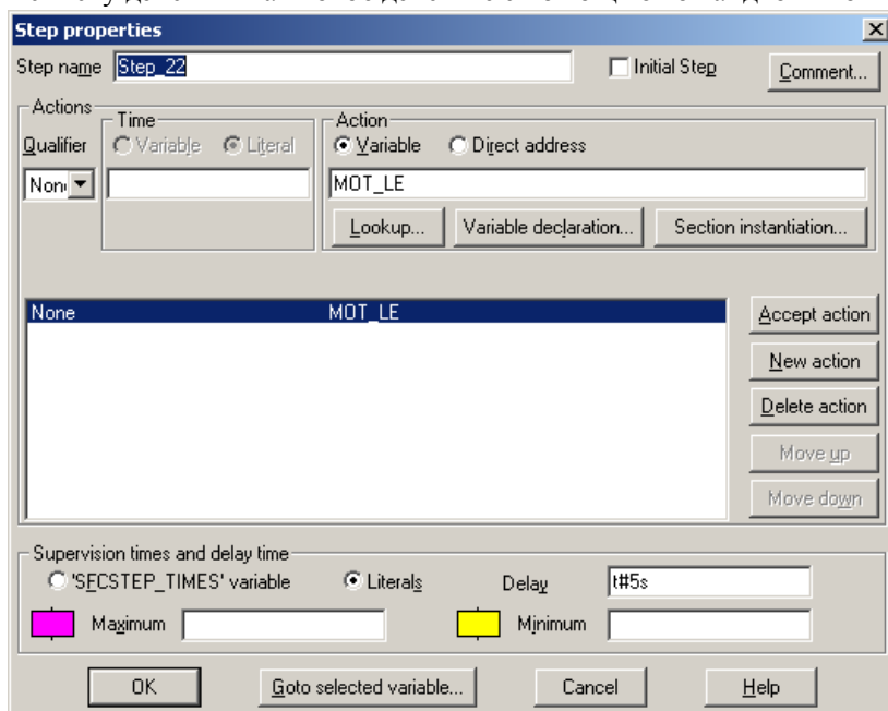
Рисунок 12 – Окно реквизитов шага
