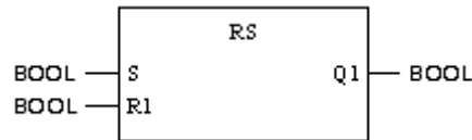
Рисунок 2 – Общий вид блока RS
