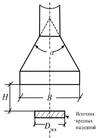
Рисунок 2 – Схема вытяжного зонга
