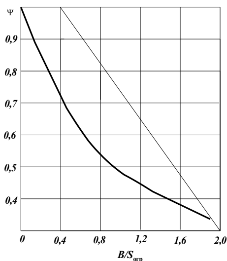
Рисунок 1 – Зависимость коэффициента диффузии \psi от постоянной помещения B и площади ограждения S_{огр}
